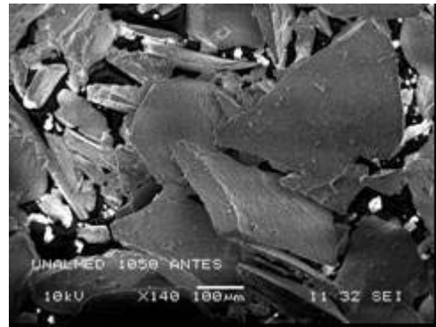
Figura 14. SEM para la muestra tratada a 1050 °C antes de la disolución.
