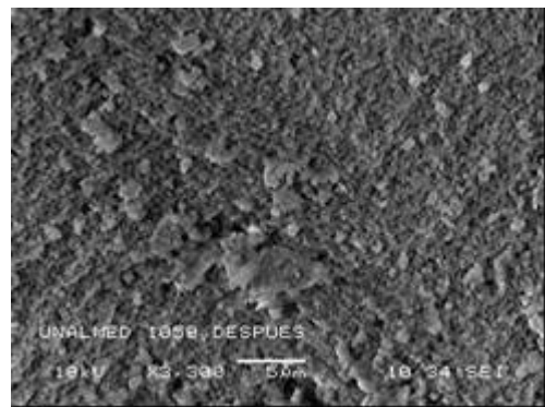
Figura 15. SEM para la muestra tratada a 1050 °C después de la disolución.
