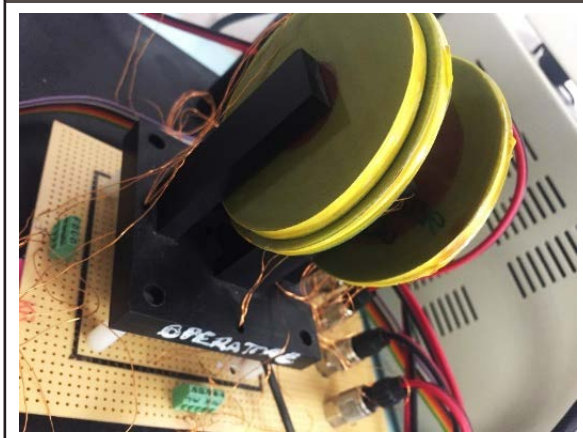
Figura 2. Sistema de electroimanes de experimentación, Instituto de Biorrobótica.
